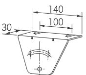
スタンド上(BZ0649)
