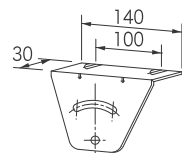
標準スタンド下(BZ0623)
