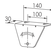
標準スタンド下(BZ0628U)
