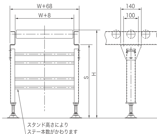
標準スタンド下(BZ0628U)
