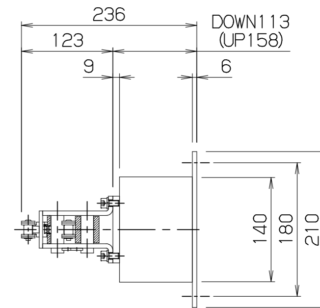
A-A断面図
