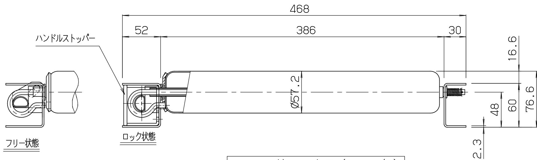
ハンドル付ローラ組図 (S=1/3)
