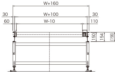
<NPA7635> <NPAU7635>( )寸法
